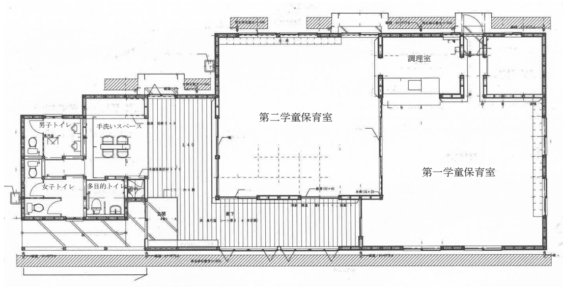
狭山市立水富小第一・第二学童保育室 平面図
