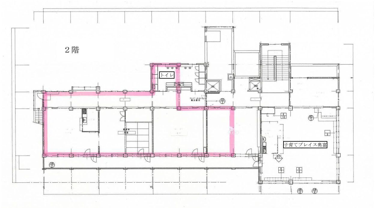
狭山市立奥富学童保育室 平面図
