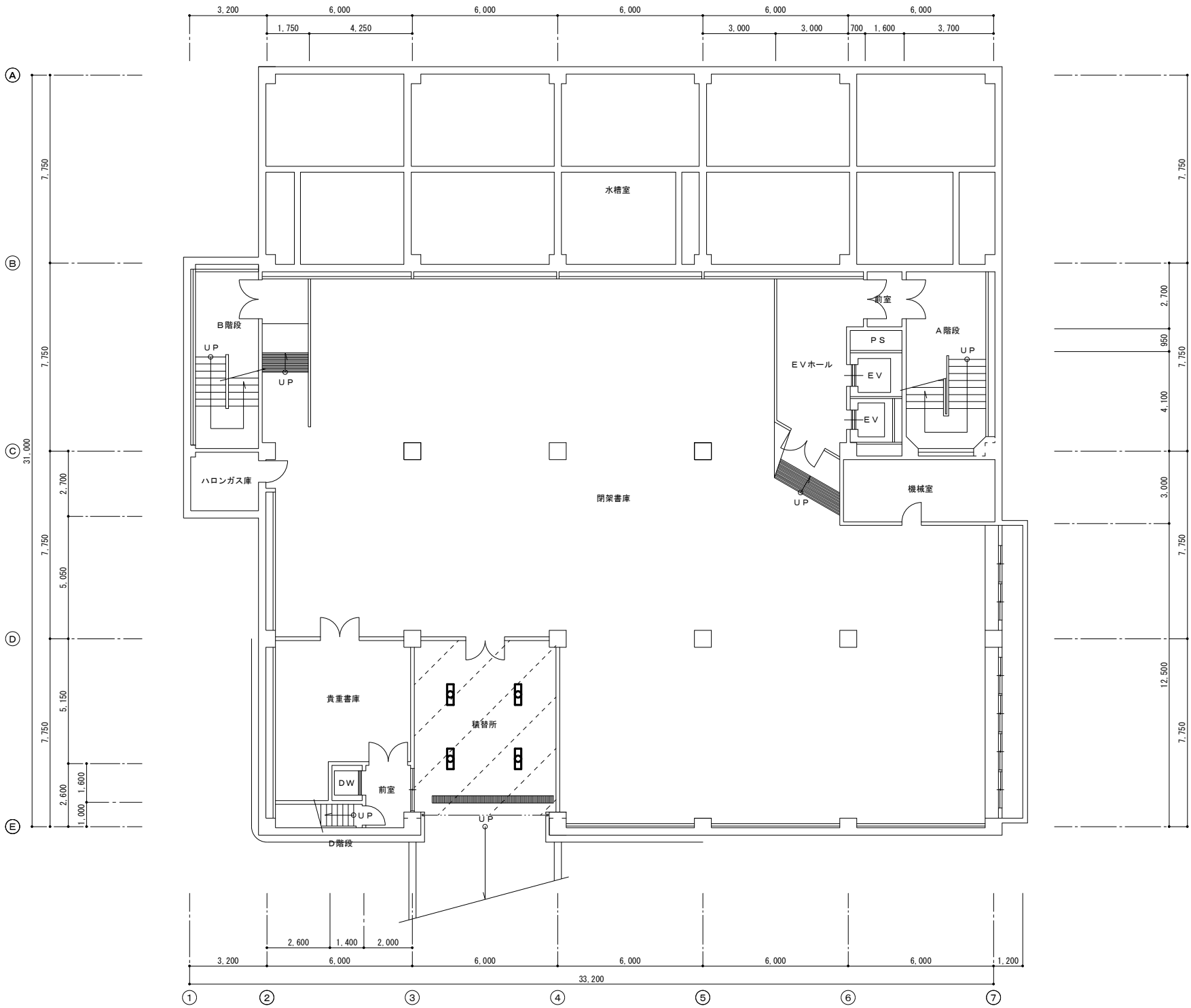
1階平面図 1/150
