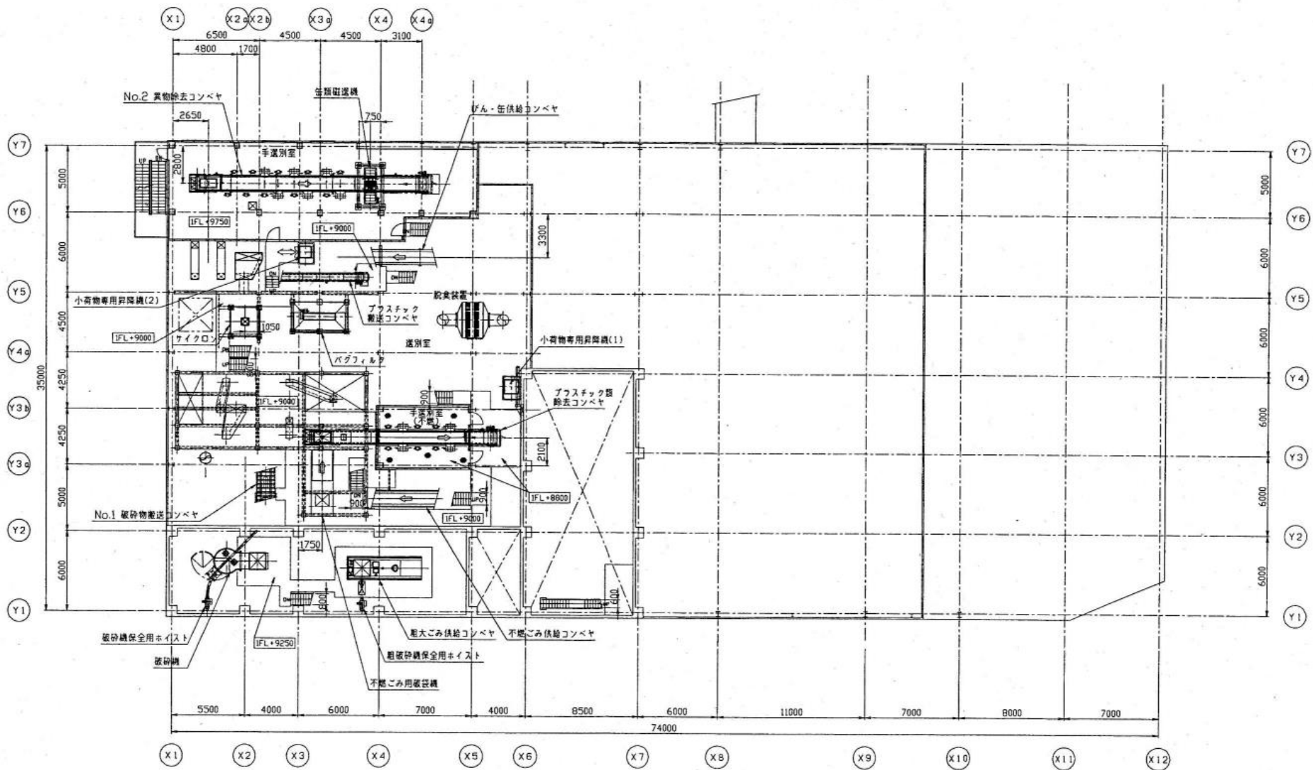
2階上部平面図
