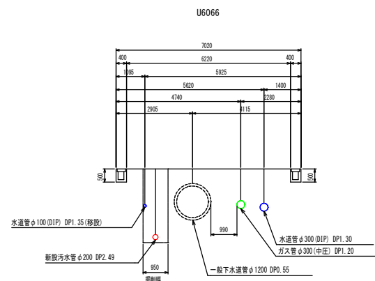
横断図 縮尺1:100
