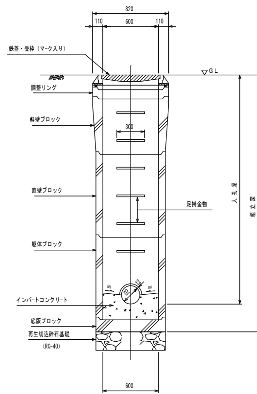
D - D 断面図
