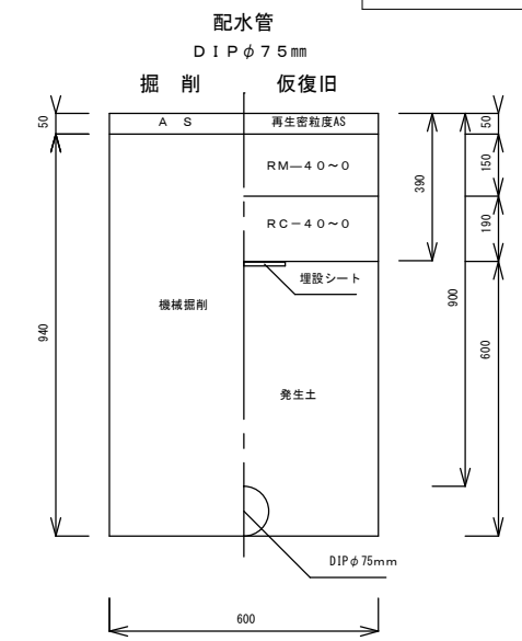
道路復旧図
