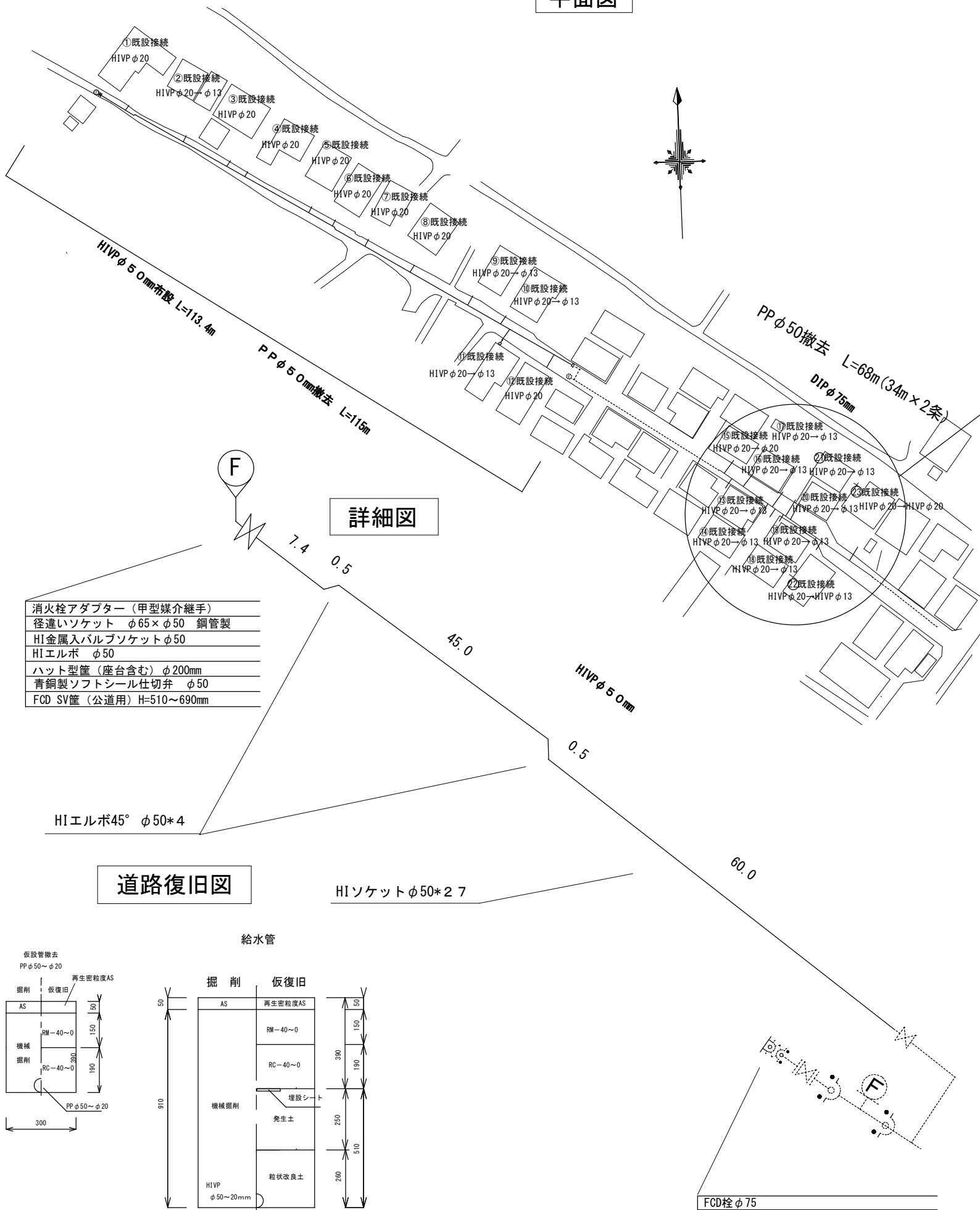
平面図
