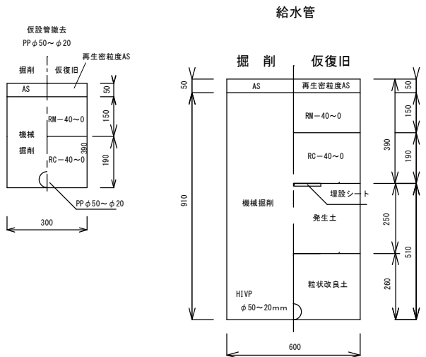
道路復旧図
