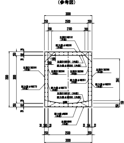
既設管渠断面図 縮尺 1:100
