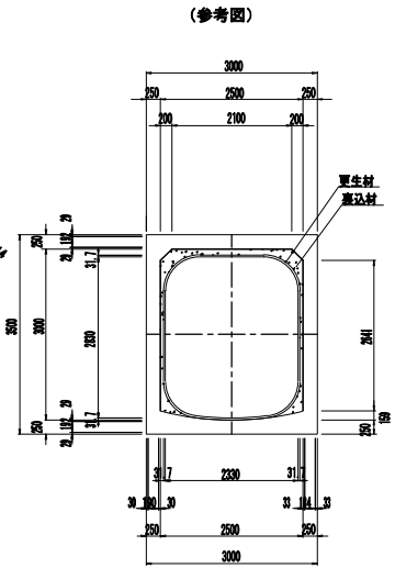
管渠更生断面図 縮尺 1:100
