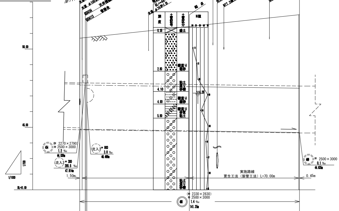
縦断面図 縮尺 縦 1:100 横 1:1000
