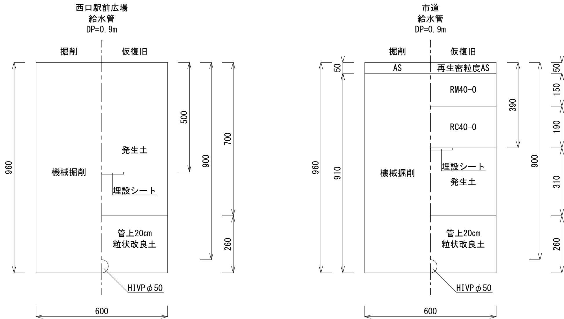
道路組成図 S=1:10
