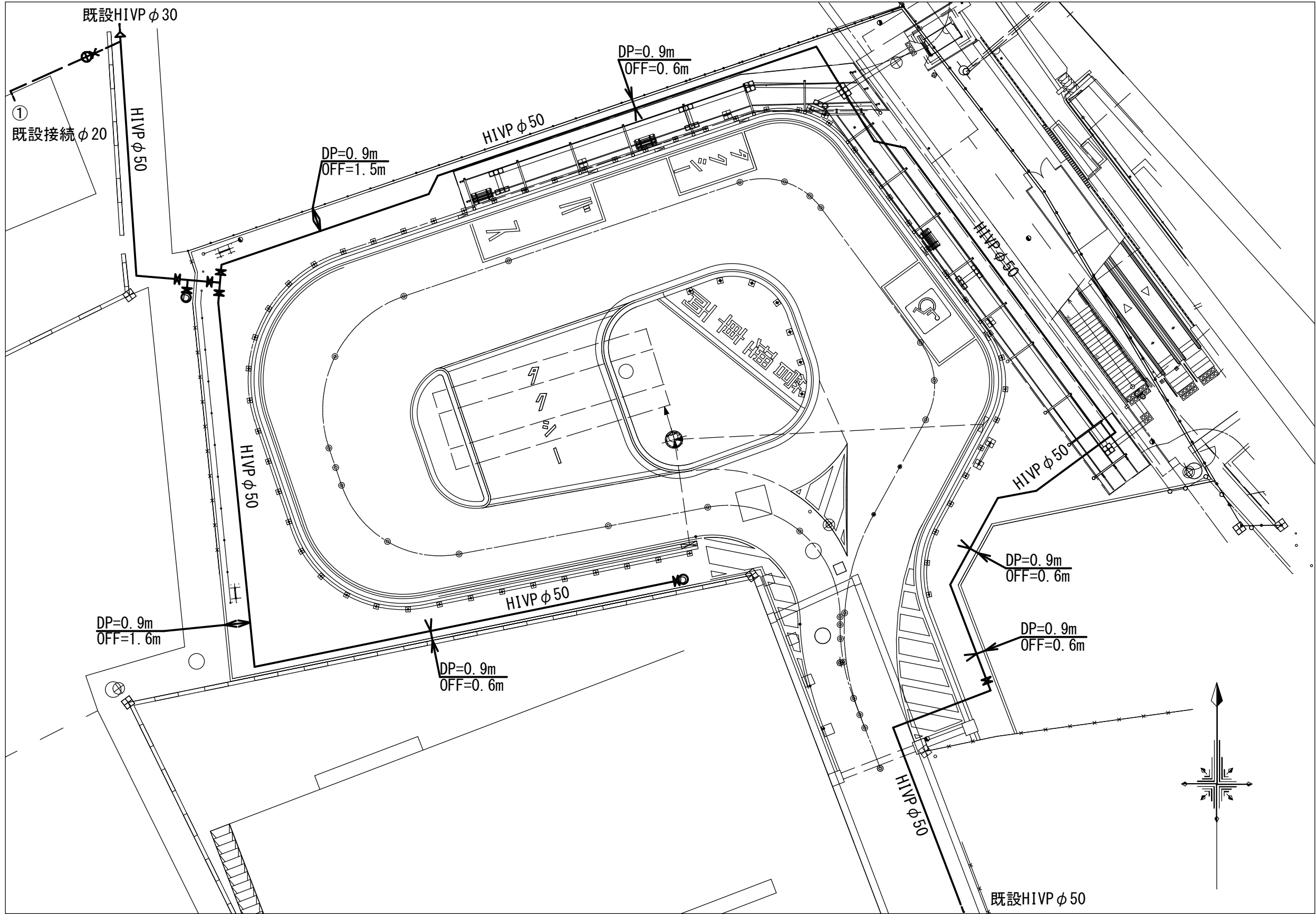
平面図 S=1:250
