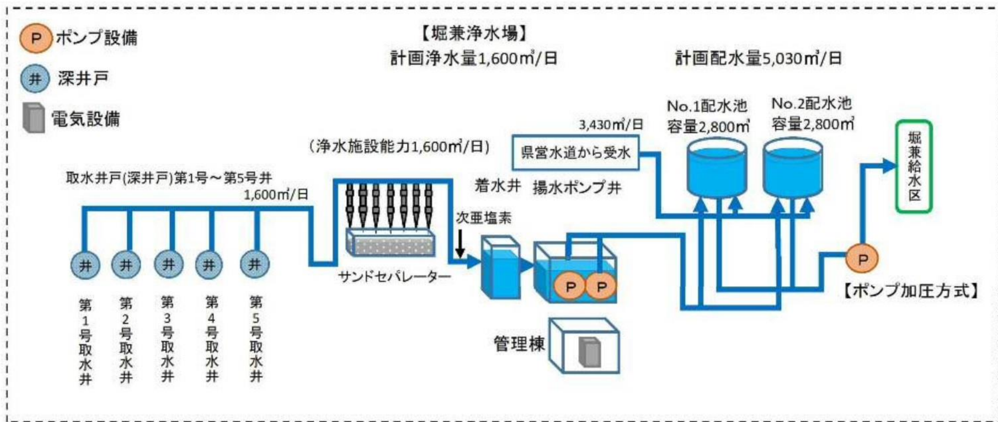
堀兼浄水場概念図
