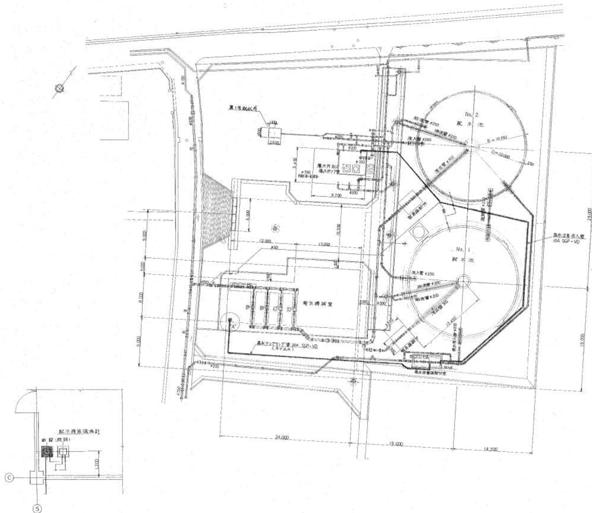
場内配管平面図 S-1:200
