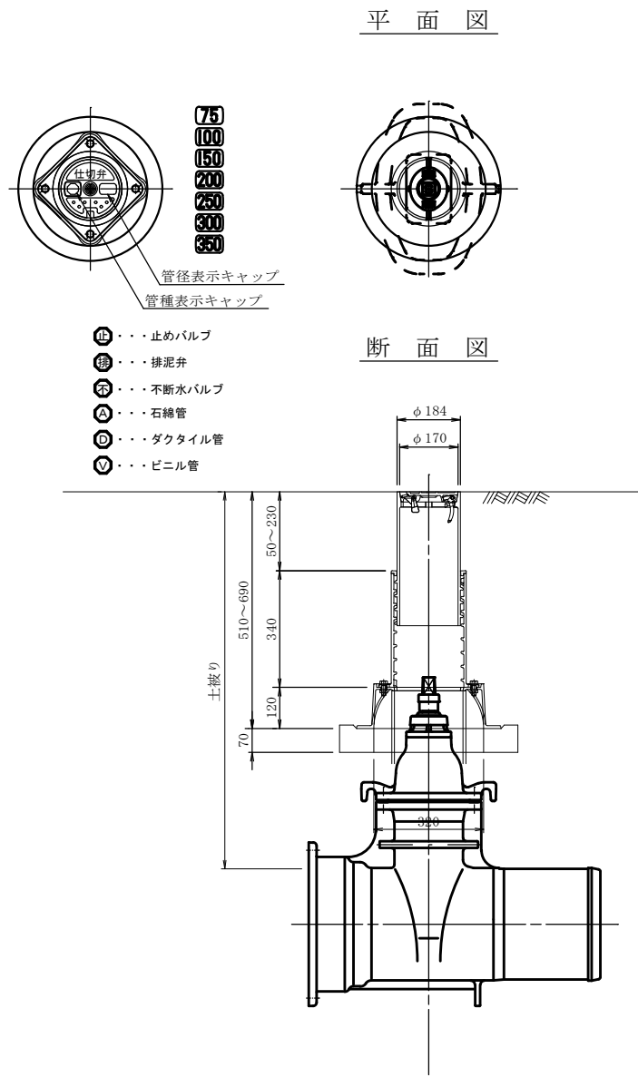
仕切弁設置標準図 S=1/10
