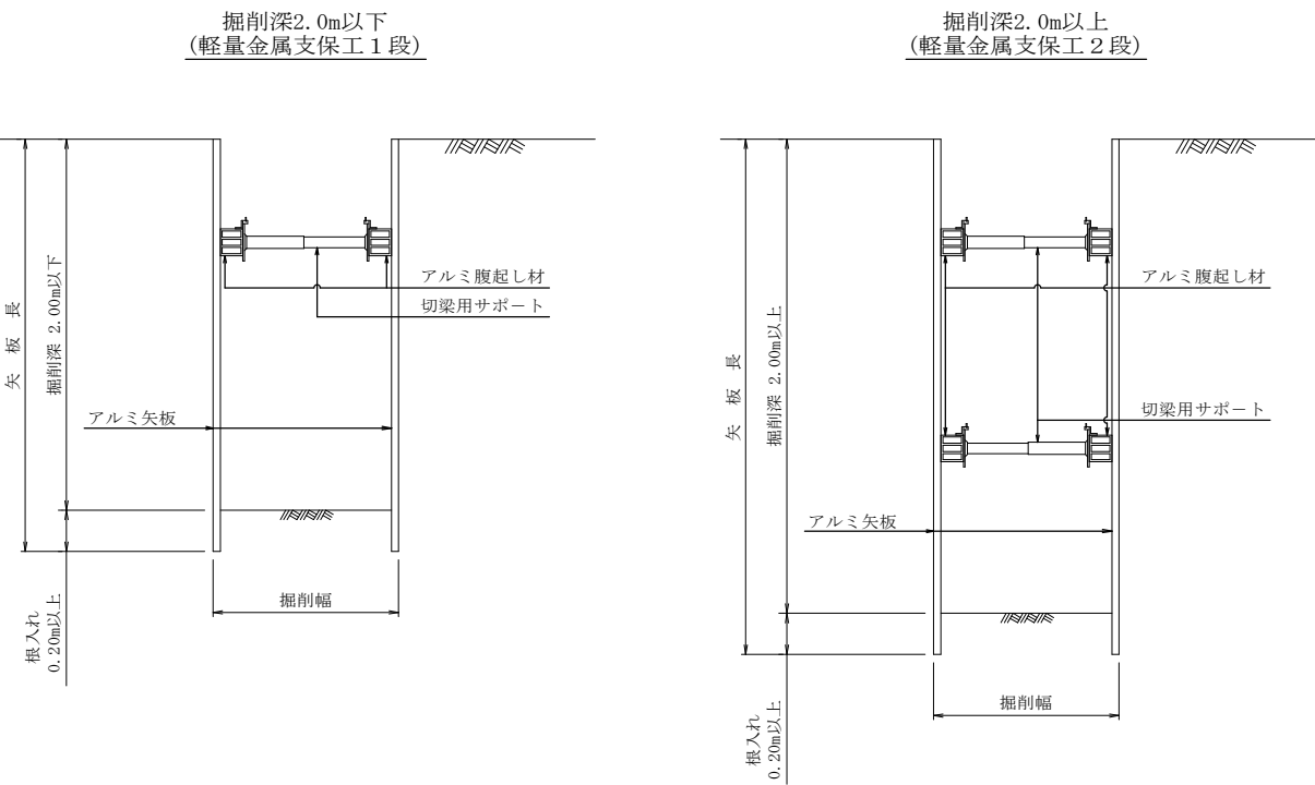
土留工標準図 S=1/20
