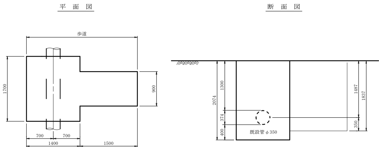
不断水割T字管土工図 S=1/30
