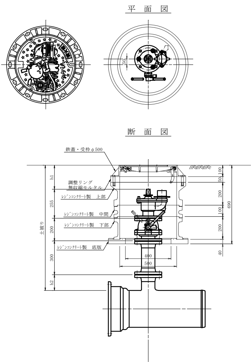
消火栓設置標準図 S=1/10
