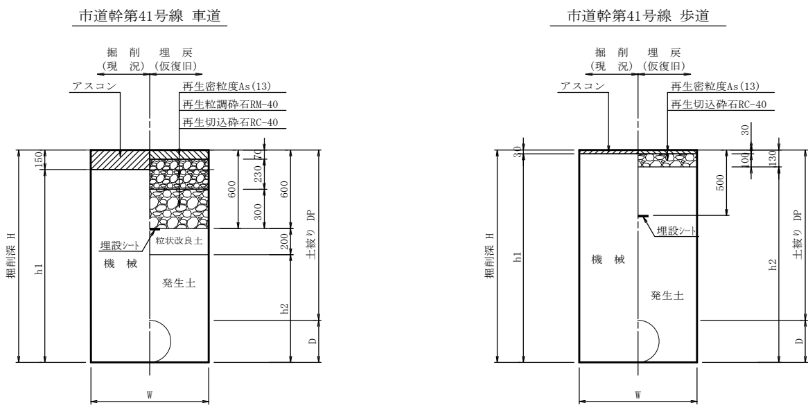
土工図及び道路復旧図 S=1/20
