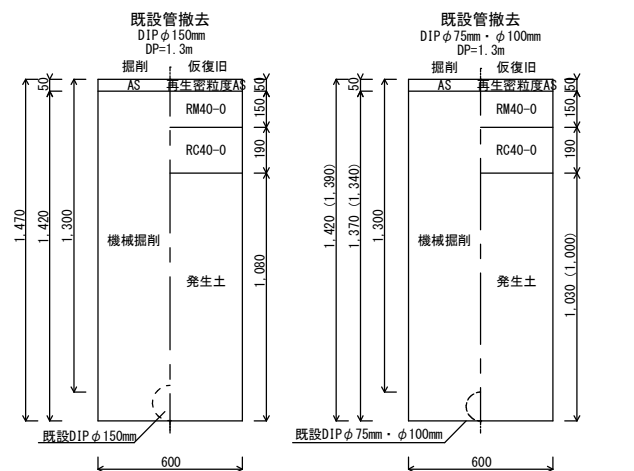
配水管撤去
