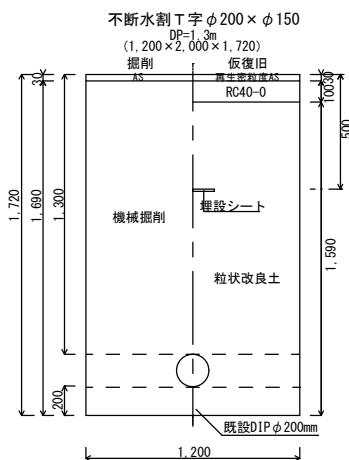
不断水割T字管 ①
