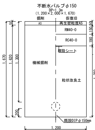
不断水バルブ ①-1
