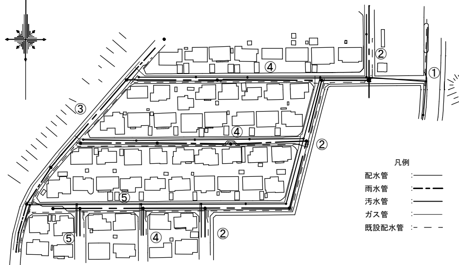
平面図 Scale:free
