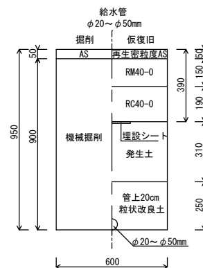
給水管
