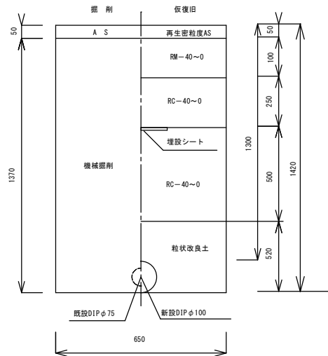
配水管（既存道路） DIPφ100設置 DIPφ75撤去
