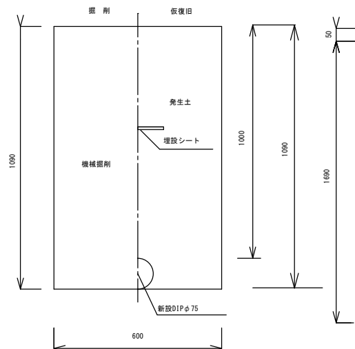
配水管（宅地内） DIPφ75設置
