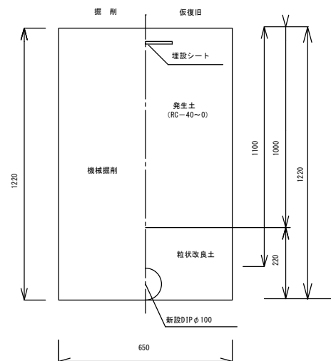
配水管（新設道路） DIPφ100設置
