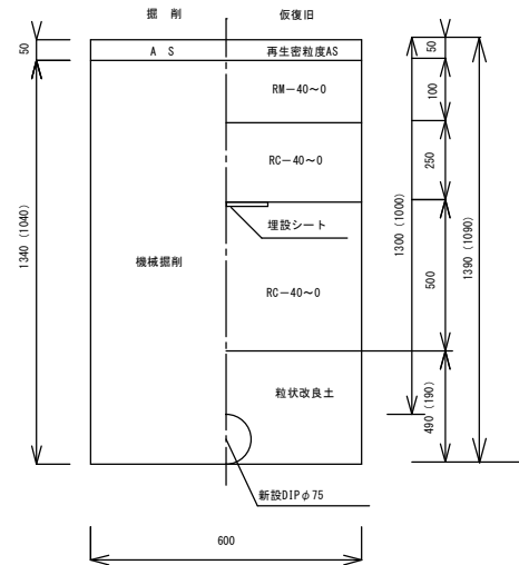
配水管（既存道路） DIPφ75設置 DP:1300 (DP:1000)
