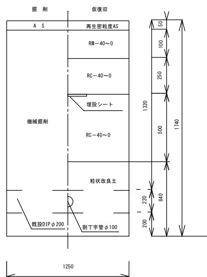
不断水割丁字 DIPφ200×φ100 (1250×1740×1500)
