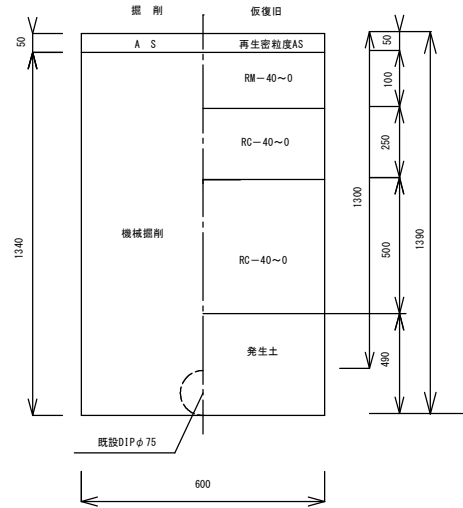
配水管（既存道路） DIPφ75撤去
