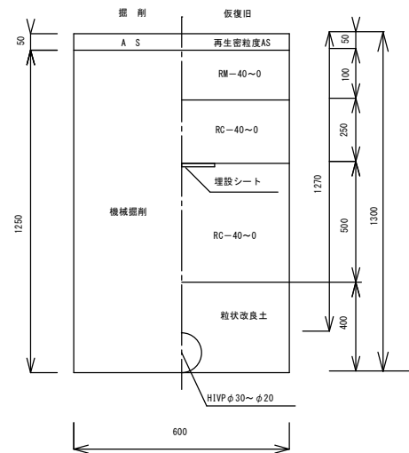
仮設給水管接続箇所 HIVPφ30~φ20 1300×600×1000
