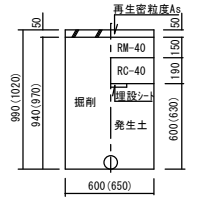
⑦⑧補強材設置DIPφ75(100) DP: 900
