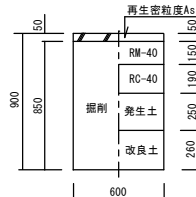
⑨給水管布設φ20~φ50 掘削深: 900
