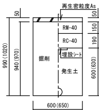
①②配水管布設DIPφ75(100) DP: 900
