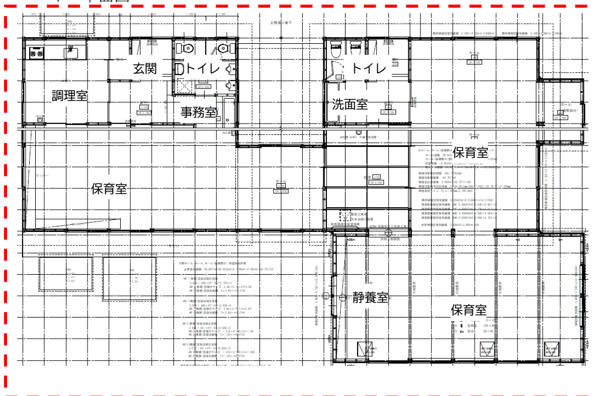
イ 平面図
