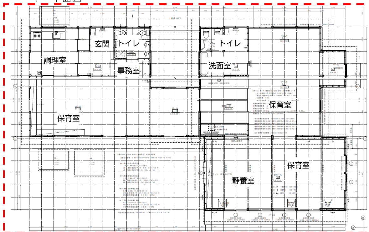
イ 平面図
