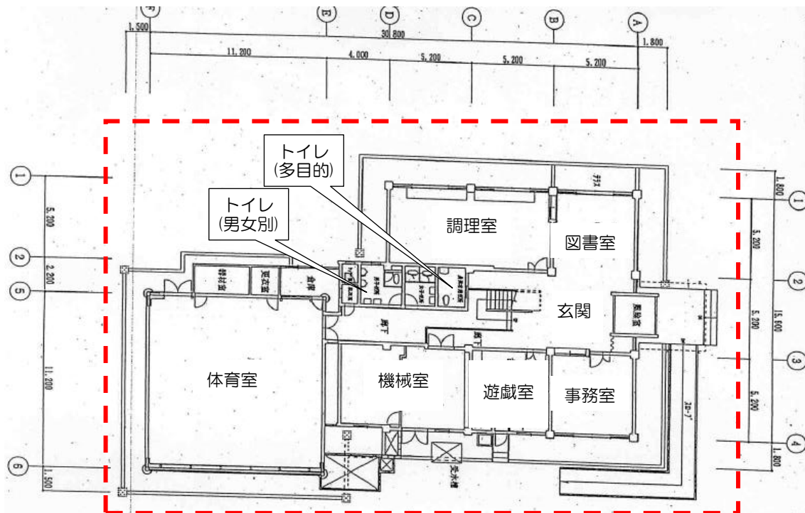
(3) 平面図 (本館 1 階)
