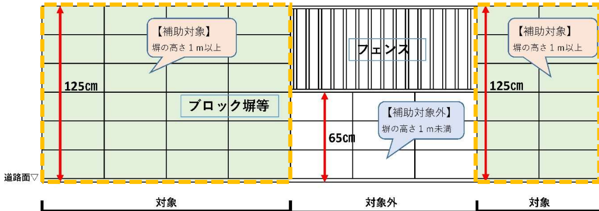
○例1 ブロック塀で一部フェンスがある場合
