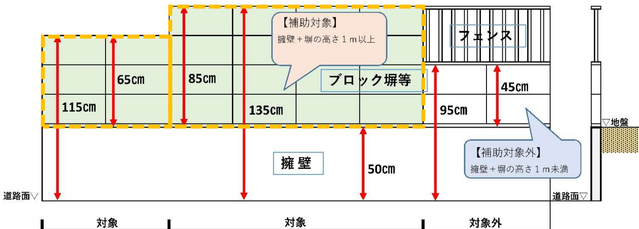
○例3 擁壁の上のブロック塀の場合
