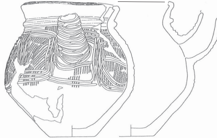
稲荷上遺跡 第56号住居跡出土土器実測図 (スケール：1/4)
