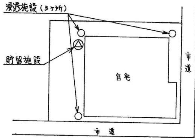
配置図 (例)
