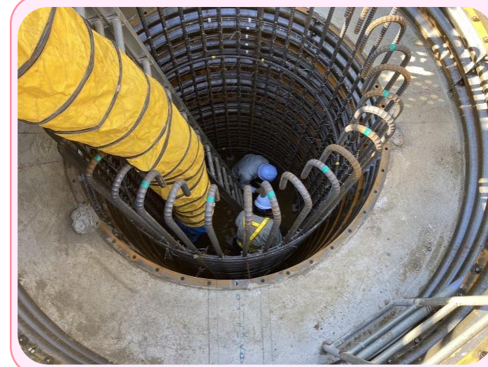
基礎杭を複数設置し入曽駅（新駅舎）を支えます
