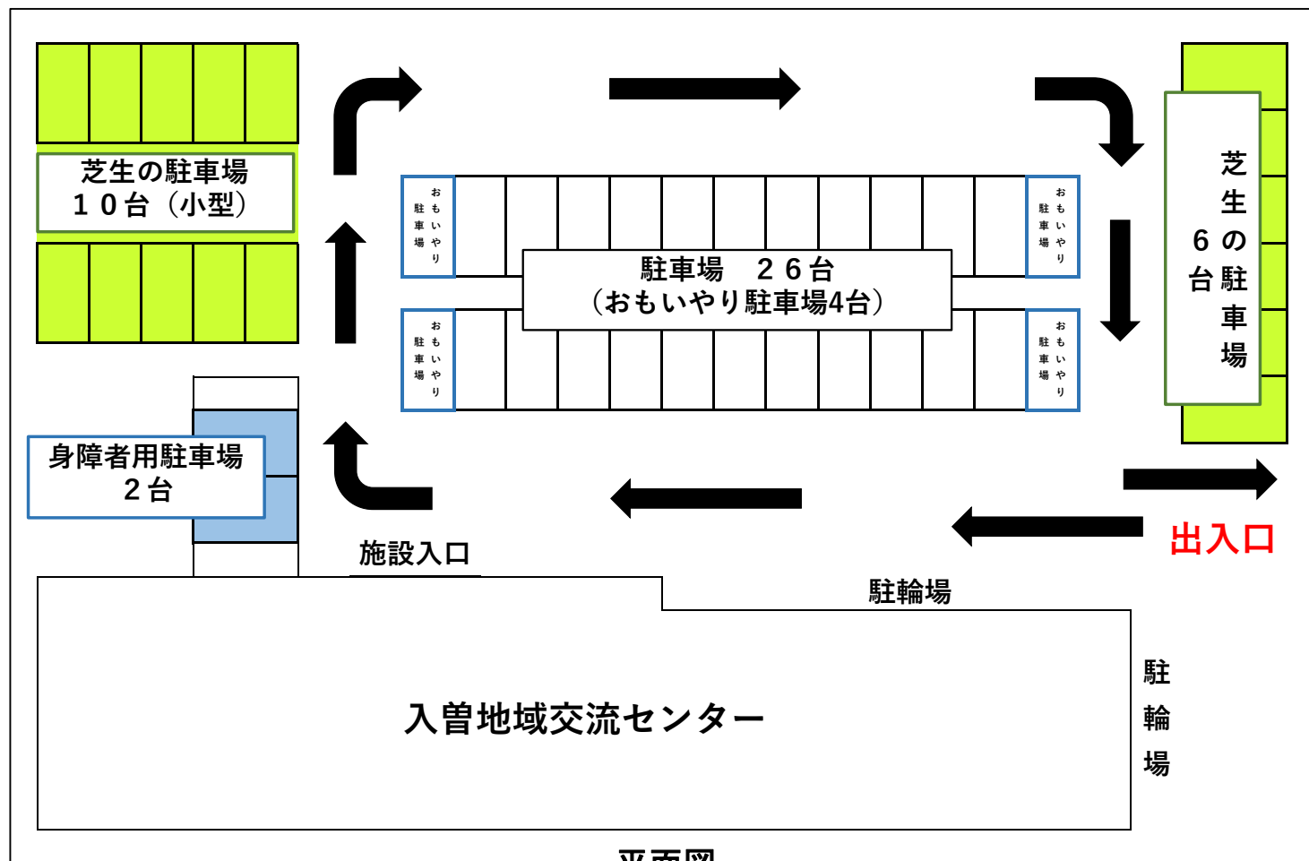
平面図
